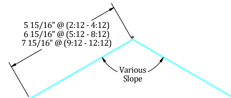
(630.2TO/UO/VO) Ridge Splice
