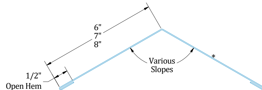
(630.3U/V/W) Hip Cap
