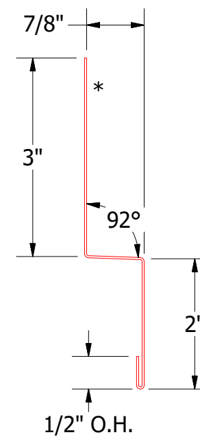
MFA550 - Head Trim
