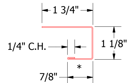
VSA118-J Channel
