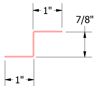
VSA681-Support Z
