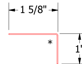
VSA680-Angle Trim
