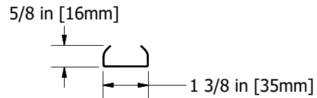
Linear Linear Ceiling (LCB138)
