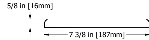
Linear Linear Ceiling (LCB738)
