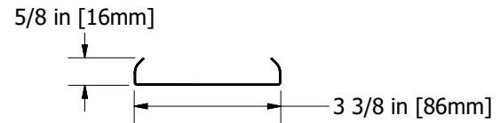
Linear Linear Ceiling (LCB338)
