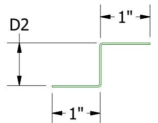
Support Z DWA681: D2 = 1" DSA681: D2 = 1 5/8"
