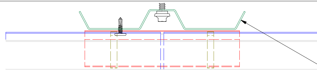
VIEW A-A
